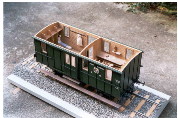
Erster Postwagen mit Innenausbau 1:10
